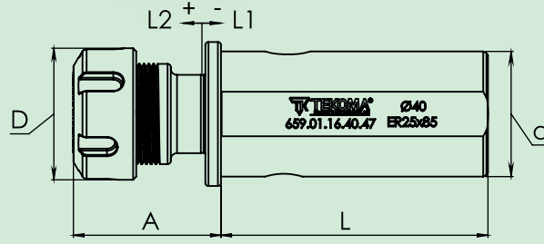
GERİ İLERİ HAREKETLİ KLAVUZ ÇEKME BAŞLIĞI
